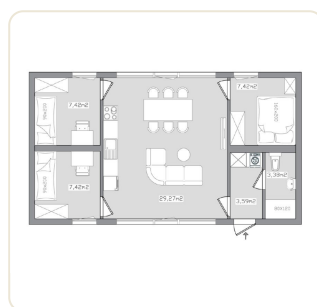
Grundriss C
