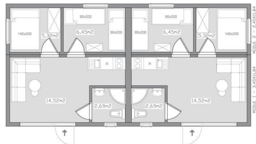
Grundriss B
