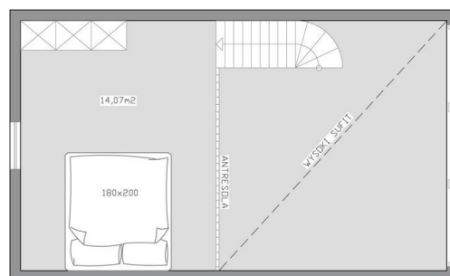
Zwischengeschoss
