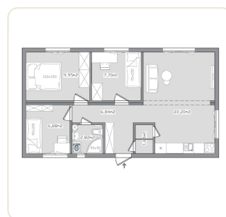
Grundriss D
